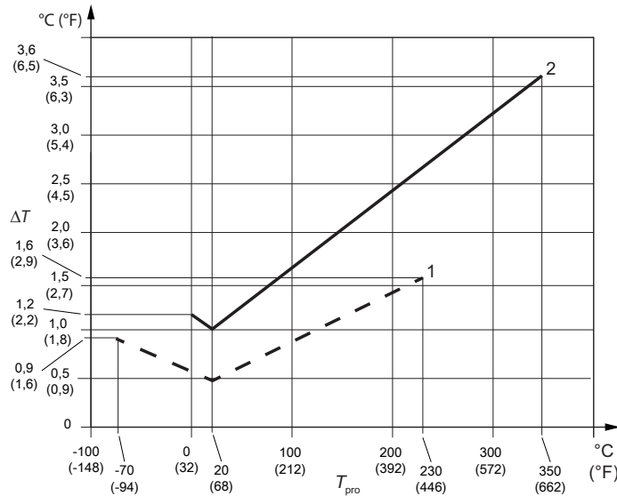
Fig. 11: Précision de température
