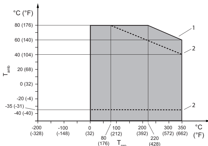
Fig. 27: Température de service du fluide à mesurer et la température ambiante admissibles, type déporté
