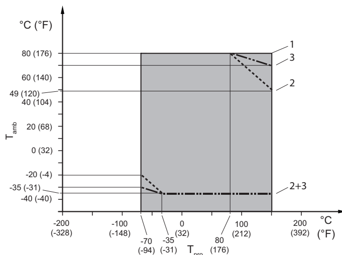
Fig. 24: Température de service du fluide à mesurer et température ambiante admissibles, type déporté (sauf pour raccordement process HS4 et HS8)
