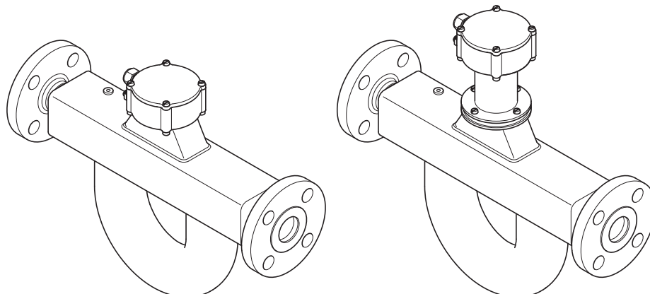
Fig. 28: Boîte de jonction standard et avec extension
