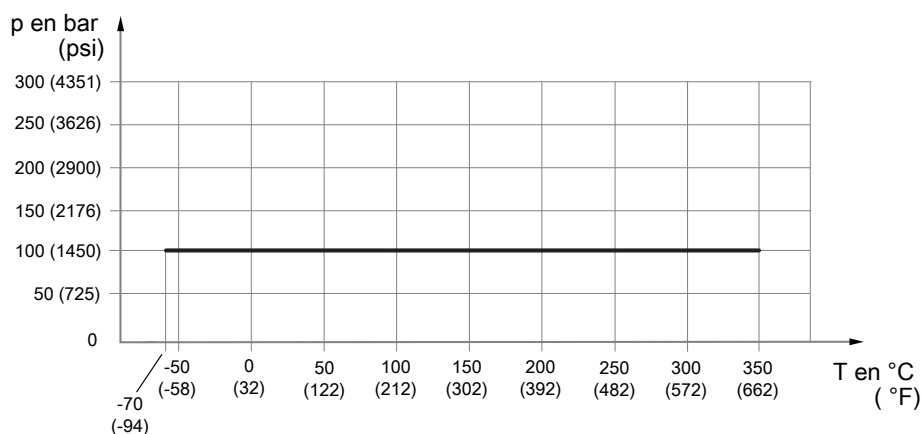
Fig. 21: Pression de service admissible en fonction de la température du raccordement process
