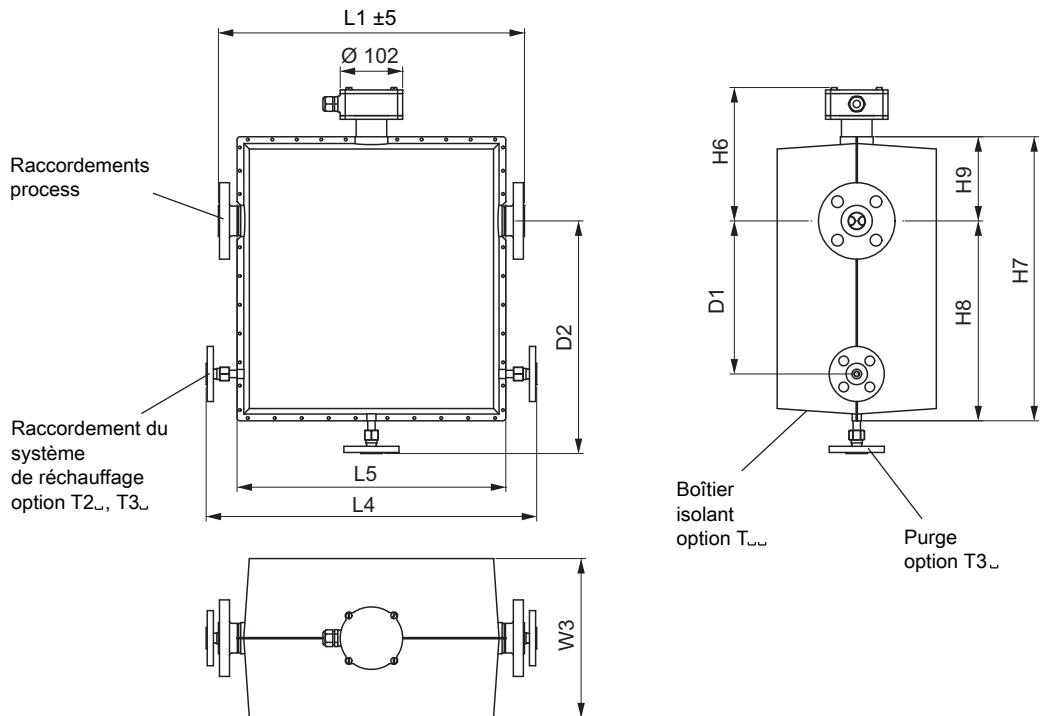
Fig. 30: Dimensions en mm : variante avec boîtier isolant
