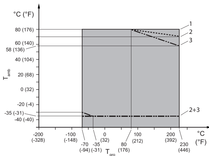
Fig. 26: Température de service du fluide à mesurer et la température ambiante admissibles, type déporté
