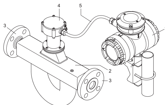
Fig. 7: Configuration du Rotamass type déporté - avec boîte de jonction avec extension
