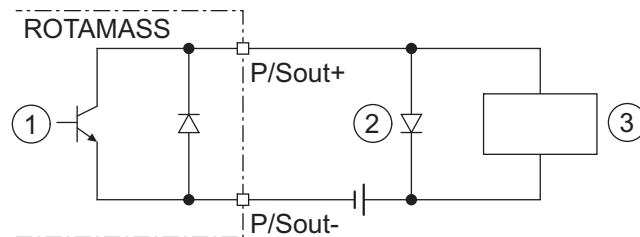
Fig. 40: Raccordement de la sortie d'impulsion passive P/Sout avec compteur électromécanique
