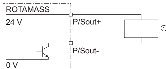
Fig. 41: Raccordement de la sortie d'état active P/Sout
