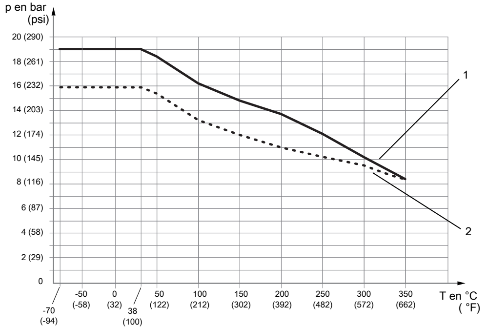
Fig. 13: Pression de service admissible en fonction de la température du raccordement process
