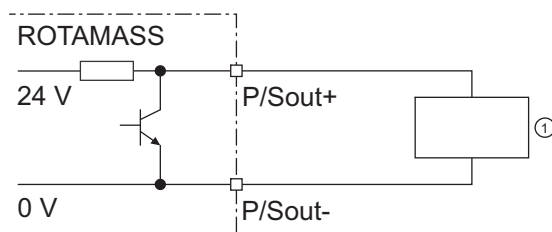
Fig. 38: Sortie d'impulsion active P/Sout avec résistance interne pull-up
