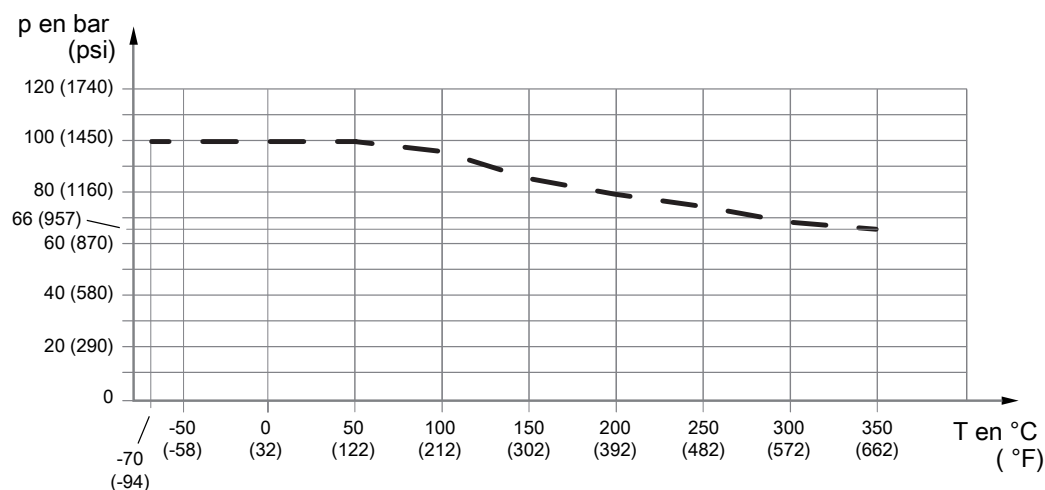
Fig. 16: Pression de service admissible en fonction de la température du raccordement process, avec bride selon EN 1092-1 PN100
