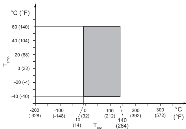
Fig. 23: Températures ambiantes et de service admissibles du fluide à mesurer, type intégral pour raccordement process HS4 et HS8
