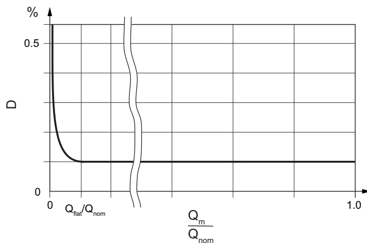
Fig. 10: Dépendance schématique de la précision de mesure du débit massique
