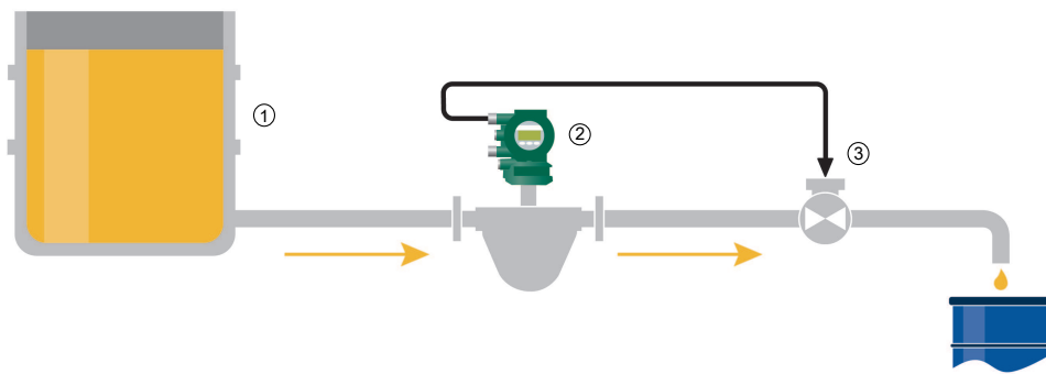
Fig. 52: Mode en une seule étape (le schéma ci-dessus illustre les fonctionnalités fondamentales pour l'une des nombreuses possibilités de combinaisons)
