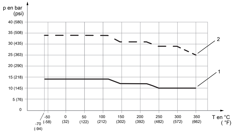
Fig. 17: Pression de service admissible en fonction de la température du raccordement process
