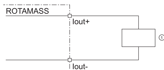
Fig. 33: Raccordement de la sortie de courant active HART lout
