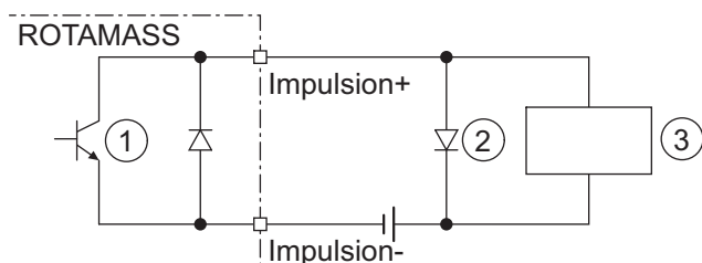
Fig. 51: Raccordement de sortie d'impulsion passive avec compteur électromécanique
