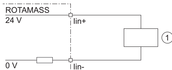
Fig. 46: Raccordement d'un appareil externe avec sortie de courant passive
