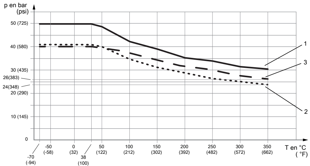
Fig. 14: Pression de service admissible en fonction de la température du raccordement process
