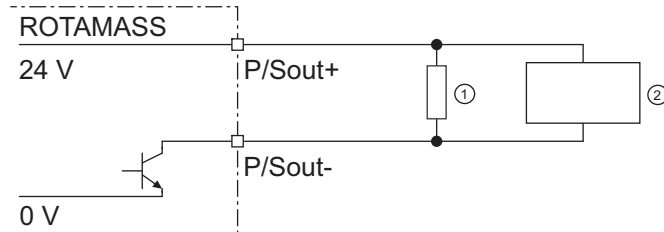
Fig. 36: Raccordement de la sortie d'impulsion active P/Sout
