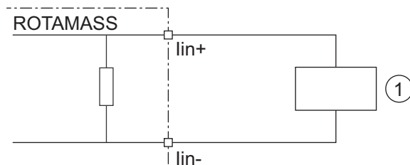
Fig. 47: Raccordement d'un appareil externe avec sortie de courant active
