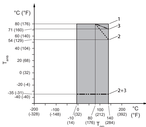
Fig. 25: Température de service du fluide à mesurer et température ambiante admissibles, type déporté pour raccordement process HS4 et HS8
