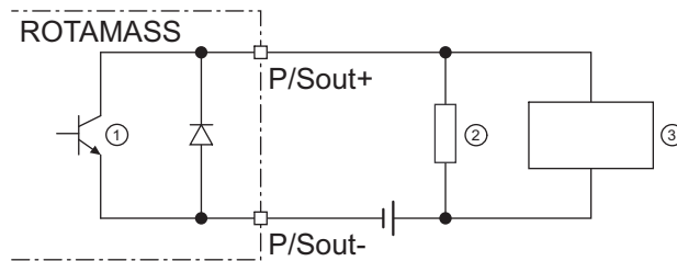
Fig. 39: Raccordement de sortie d'impulsion passive P/Sout avec compteur électronique
