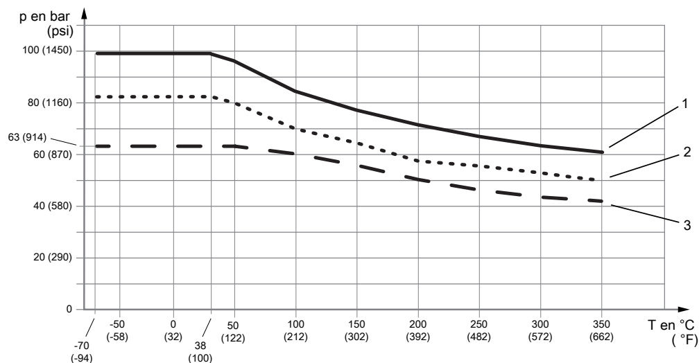
Fig. 15: Pression de service admissible en fonction de la température du raccordement process
