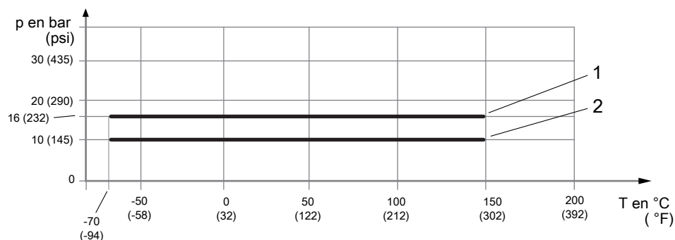
Fig. 20: Pression de service admissible en fonction de la température du raccordement process
