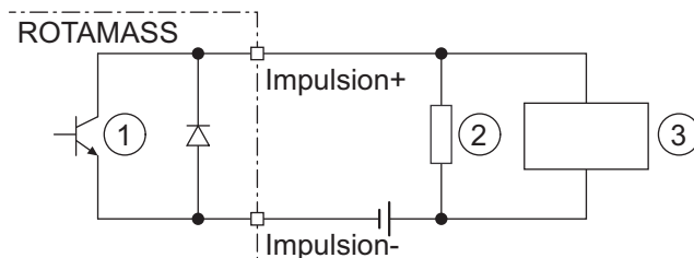
Fig. 50: Raccordement de sortie d'impulsion passive avec compteur électronique
