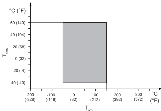
Fig. 22: Température de service du fluide à mesurer et température ambiante admissibles, type intégré (sauf pour raccordement process HS4 et HS8)
