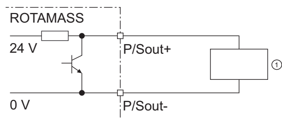
Fig. 42: Sortie d'état active P/Sout avec résistance interne pull-up
