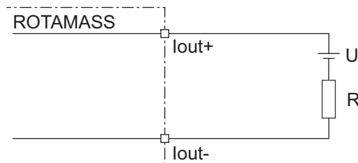
Fig. 35: Raccordement de la sortie de courant passive I out
