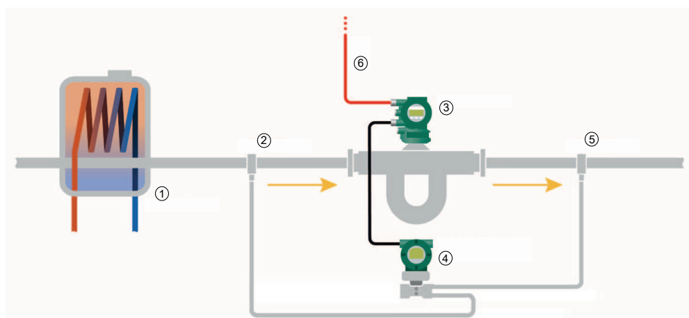
Fig. 54: Position des vannes de pression
