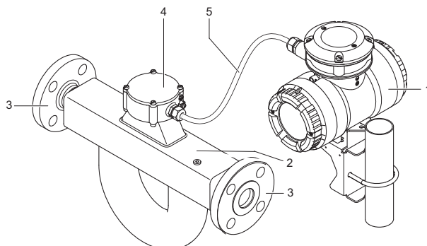
Fig. 6: Conception du Rotamass de type déporté
