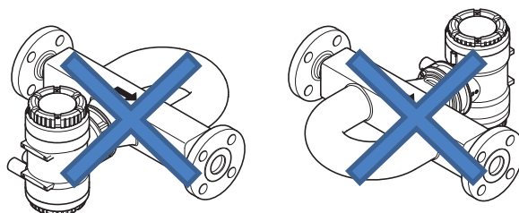
Fig. 12: Position de montage à éviter : Débitmètre en position latérale
