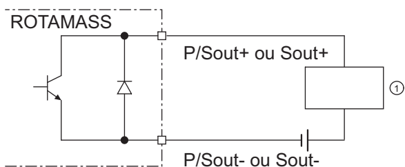
Fig. 43: Raccordement de la sortie d'état passive P/Sout ou Sout
