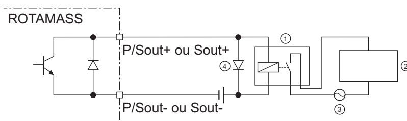
Fig. 44: Raccordement de la sortie d'état passive P/Sout ou Sout pour la commutation d'une électrovanne
