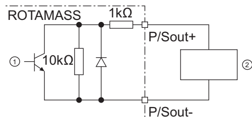
Fig. 45: Raccordement en série de la sortie d'impulsions ou d'état passive avec amplificateur de commutation
