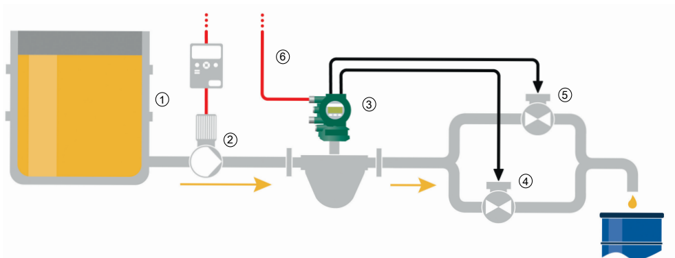
Fig. 53: Mode en deux étapes (le schéma ci-dessus illustre les fonctionnalités fondamentales pour l'une des nombreuses possibilités de combinaisons)
