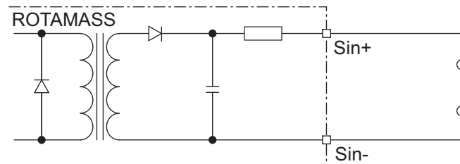
Fig. 48: Raccordement de l'entrée d'état
