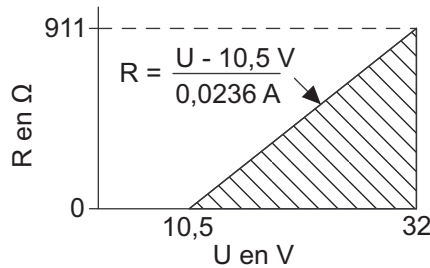
Fig. 34: Résistance de charge maximale en fonction d'une tension d'alimentation externe
