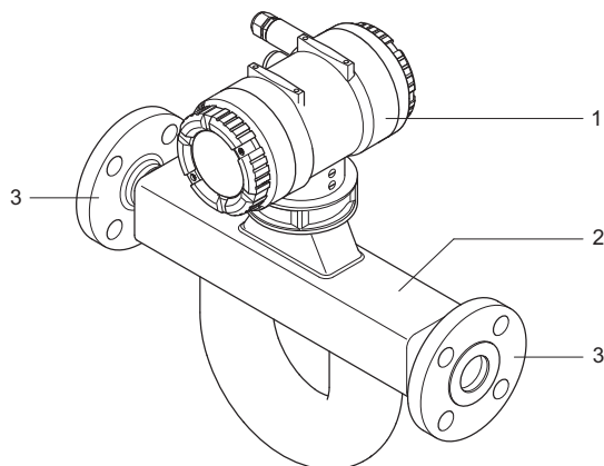
Fig. 5: Conception du Rotamass de type intégré
