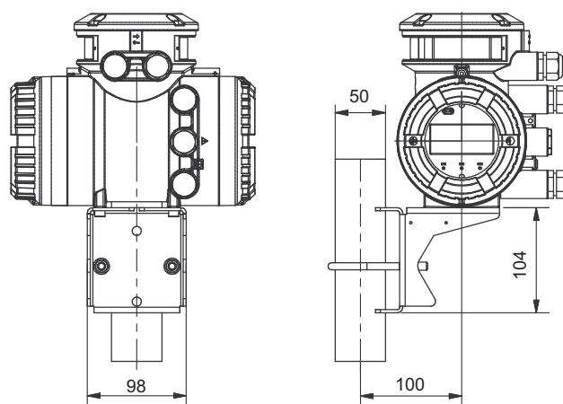
Fig. 32: Dimensions du transmetteur en mm, fixé à l'étrier de maintien
