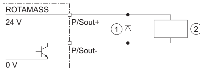
Fig. 37: Raccordement de sortie d'impulsion active P/Sout avec compteur électromécanique
