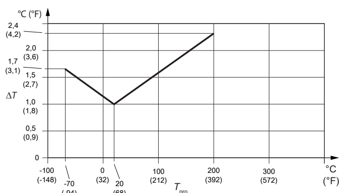
Abb. 10: Temperatur-Messgenauigkeit
