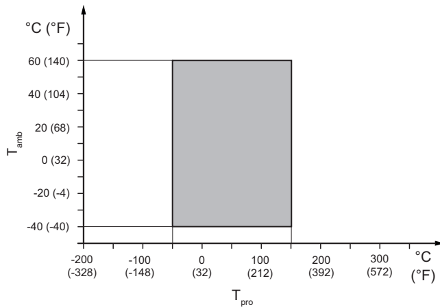
Abb. 18: Zulässige Prozess- und Umgebungstemperaturen, Kompaktausführung
