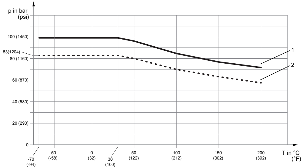
Abb. 14: Zulässiger Prozessdruck in Abhängigkeit von der Prozessanschlusstemperatur
