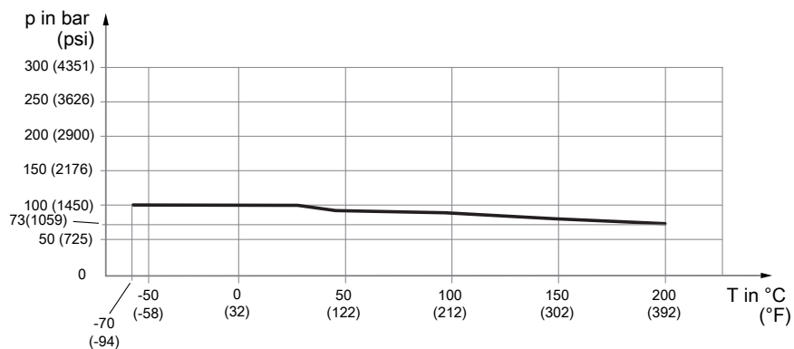
Abb. 17: Zulässiger Prozessdruck in Abhängigkeit von der Prozessanschlusstemperatur
