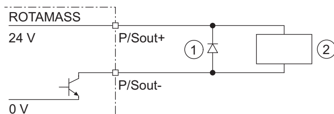
Abb. 28: Anschluss aktiver Impulsausgang P/Sout mit elektromechanischem Zähler
