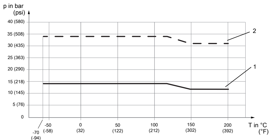
Abb. 16: Zulässiger Prozessdruck in Abhängigkeit von der Prozessanschlusstemperatur
