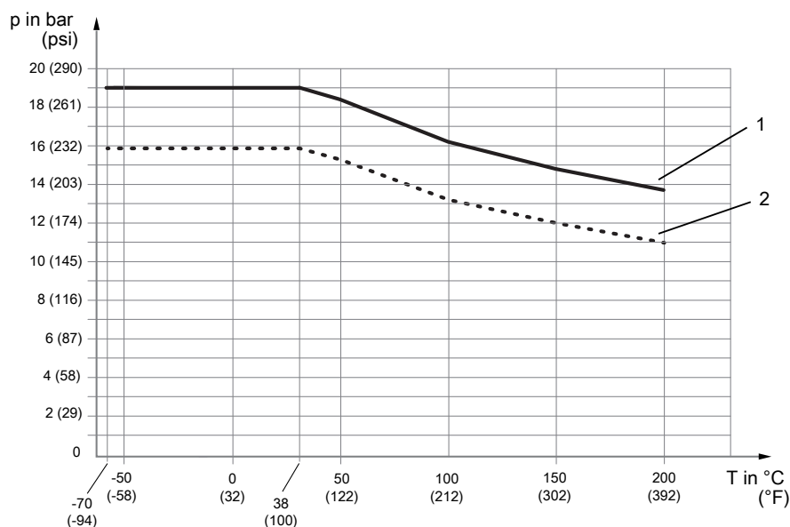
Abb. 12: Zulässiger Prozessdruck in Abhängigkeit von der Prozessanschlussstemperatur
