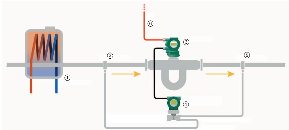
Abb. 45: Lage der Druckmessstutzen
