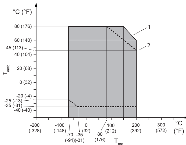
Abb. 19: Zulässige Prozess- und Umgebungstemperaturen, getrennte Ausführung
