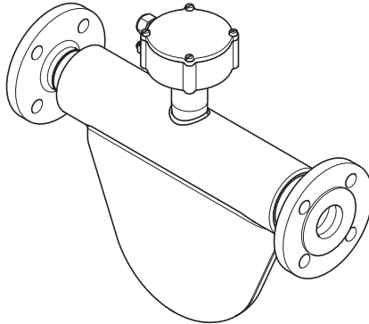
Abb. 20: Messaufnehmer getrennte Ausführung mit Standardanschlussgehäuse
