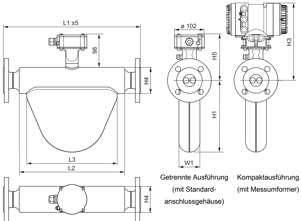
Abb. 21: Abmessungen in mm
