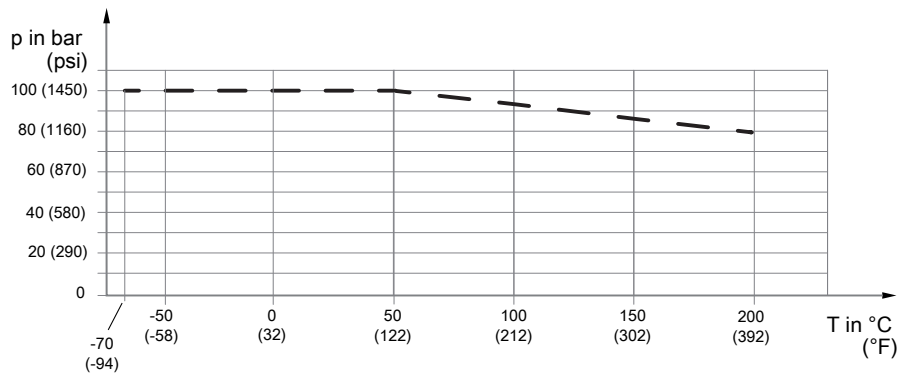
Abb. 15: Zulässiger Prozessdruck in Abhängigkeit von der Prozessanschlusstemperatur, passend zu Flansch EN 1092-1 PN100
