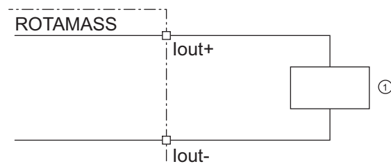
Abb. 24: Anschluss aktiver Stromausgang lout HART
