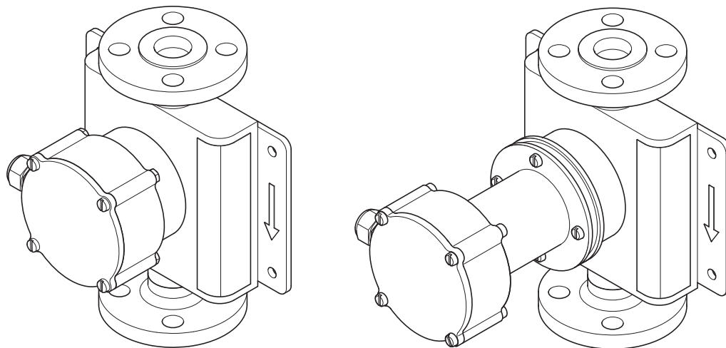
Fig. 25: Capteur avec boîte de jonction standard et avec extension
