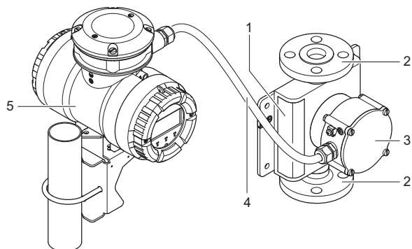
Fig. 5: Conception du Rotamass de type déporté
