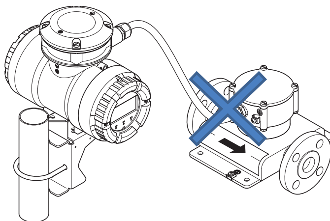
Fig. 11: Position de montage à éviter : Débitmètre en position latérale
