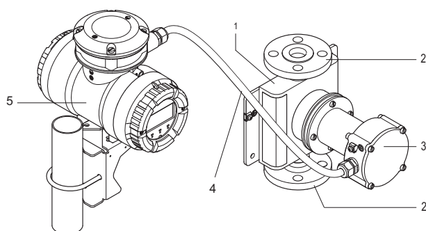
Fig. 6: Configuration du Rotamass type déporté - avec boîte de jonction avec extension
