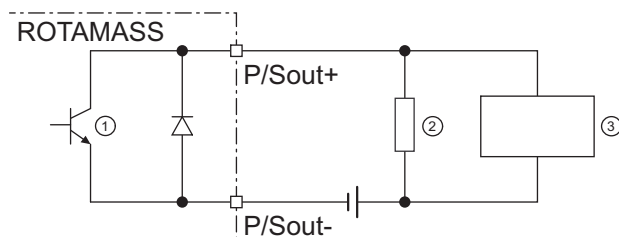
Fig. 37: Raccordement de sortie d'impulsion passive P/Sout avec compteur électronique
