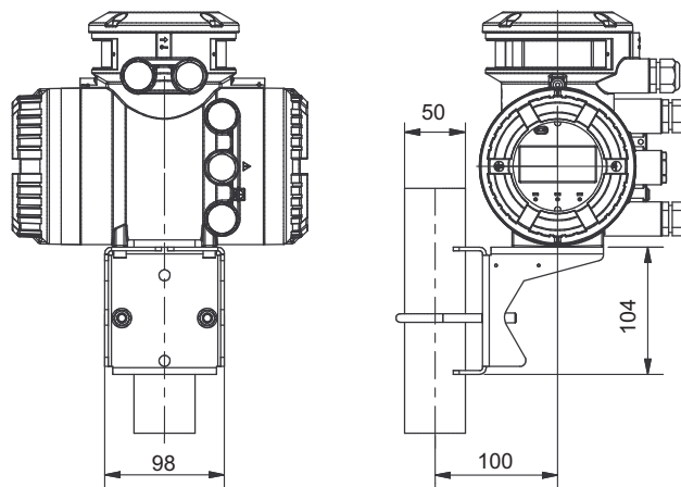
Fig. 30: Dimensions du transmetteur en mm, fixé à l'étrier de maintien
