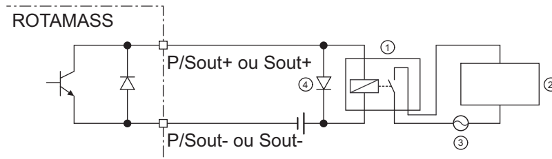
Fig. 42: Raccordement de la sortie d'état passive P/Sout ou Sout pour la commutation d'une électrovanne
