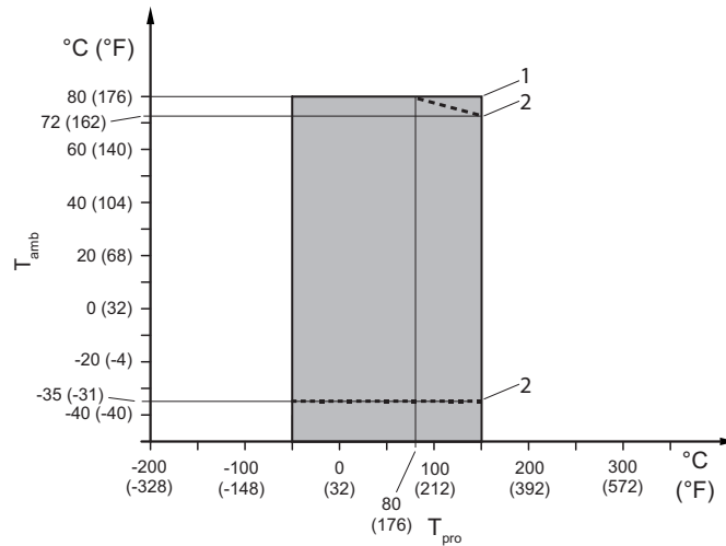
Fig. 22: Température de service du fluide à mesurer et température ambiante admissibles, type déporté (sauf pour raccordement process HS4 et HS8)
