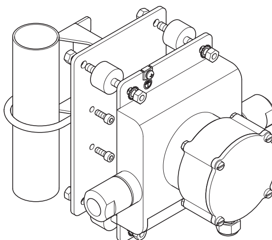
Fig. 53: Dispositif de fixation pour le capteur PD en option Rotamass Nano sensor
