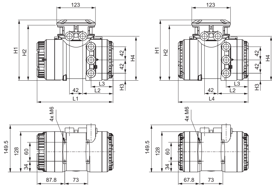
Fig. 29: Dimensions du transmetteur en mm (à gauche : transmetteur avec écran, à droite : transmetteur sans écran)
