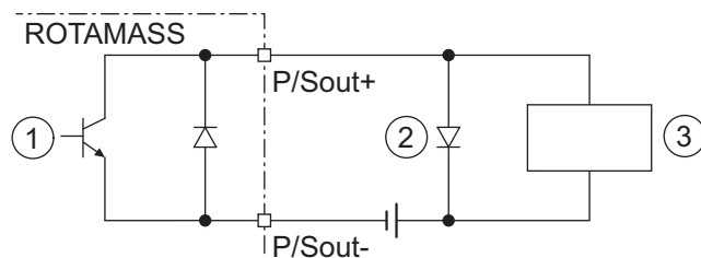
Fig. 38: Raccordement de la sortie d'impulsion passive P/Sout avec compteur électromécanique
