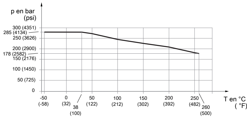
Fig. 20: Pression de service admissible en fonction de la température du raccordement process
