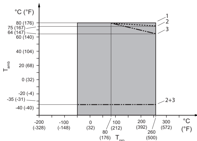
Fig. 24: Température de service du fluide à mesurer et température ambiante admissibles
