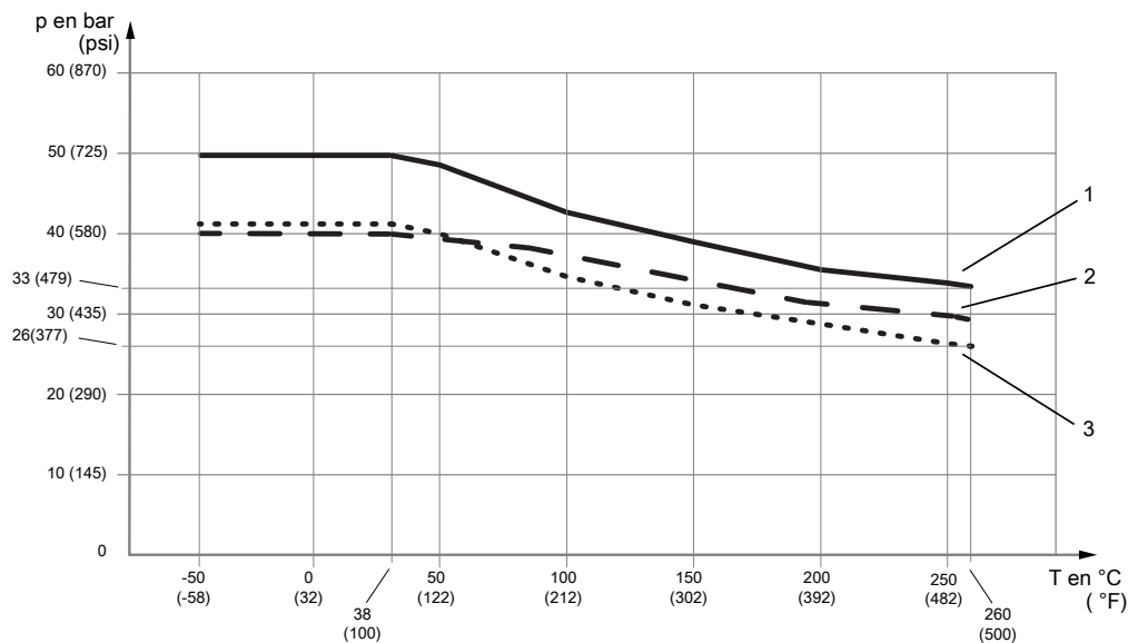
Fig. 13: Pression de service admissible en fonction de la température du raccordement process
