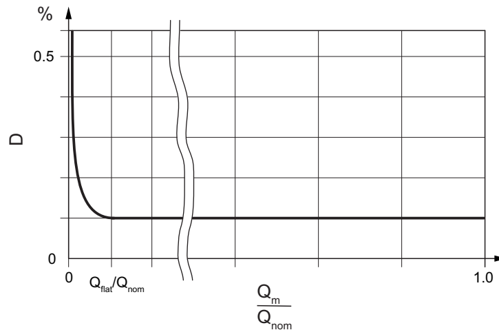
Fig. 9: Dépendance schématisée de la précision de mesure du débit massique
