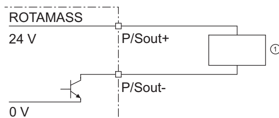
Fig. 39: Raccordement de la sortie d'état active P/Sout
