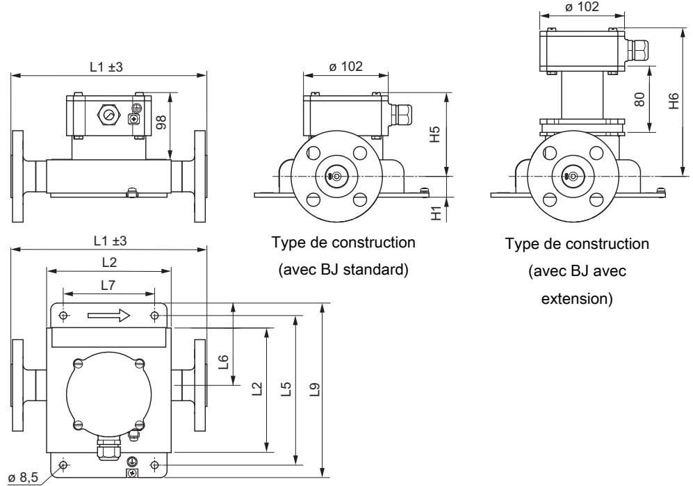
Fig. 26: Dimensions en mm
