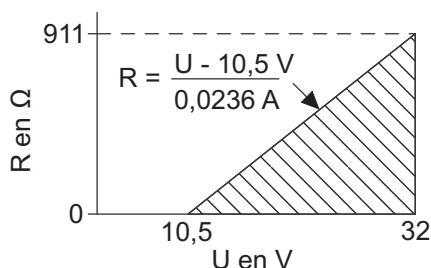
Fig. 32: Résistance de charge maximale en fonction d'une tension d'alimentation externe
