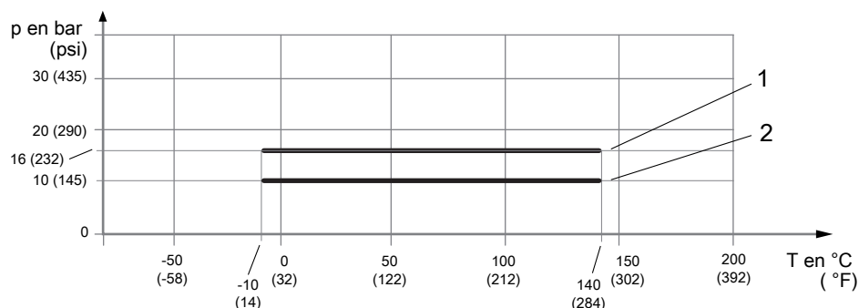
Fig. 18: Pression de service admissible en fonction de la température du raccordement process
