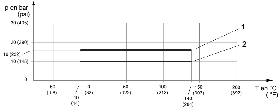
Fig. 19: Pression de service admissible en fonction de la température du raccordement process
