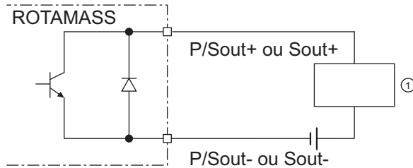
Fig. 41: Raccordement de la sortie d'état passive P/Sout ou Sout
