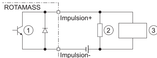
Fig. 48: Raccordement de sortie d'impulsion passive avec compteur électronique
