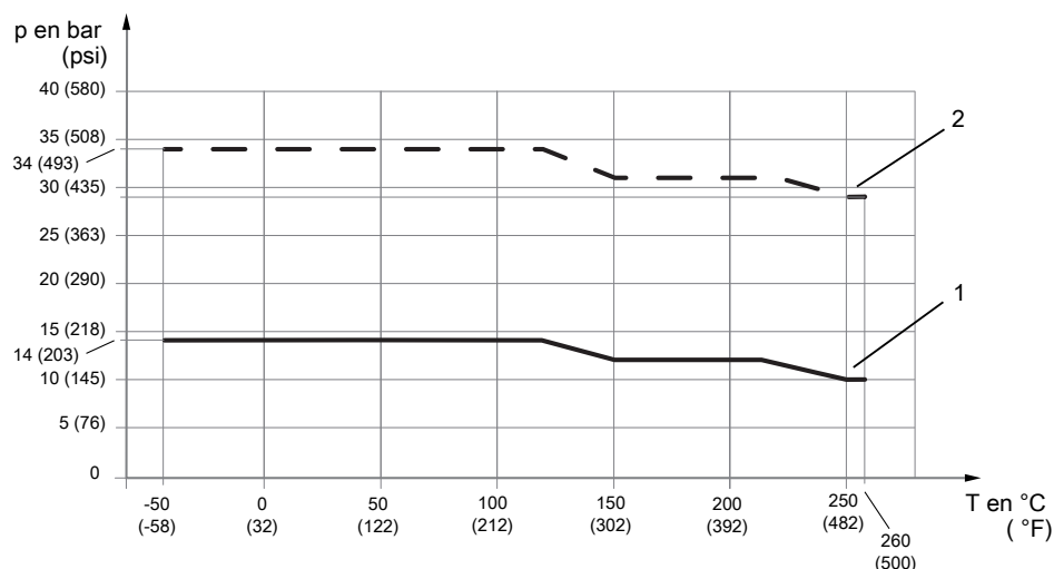
Fig. 17: Pression de service admissible en fonction de la température du raccordement process
