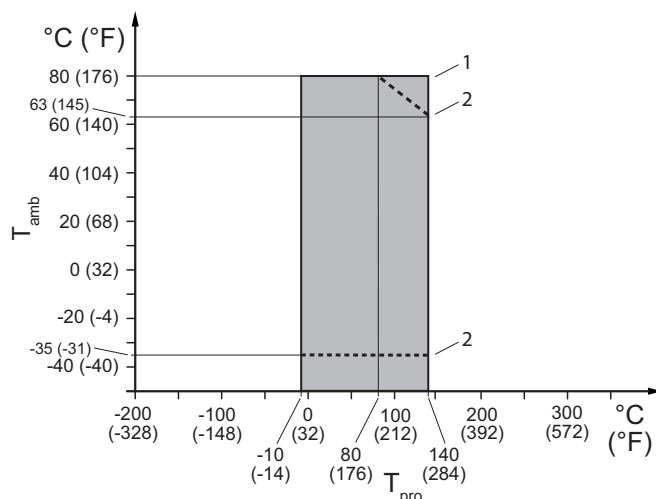
Fig. 23: Température de service du fluide à mesurer et température ambiante admissibles, type déporté pour raccordement process HS4 et HS8
