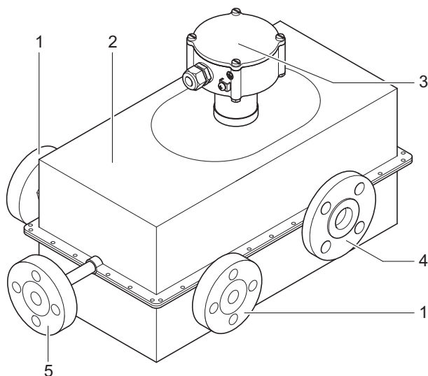
Fig. 21: Configuration du Rotamass avec isolation et circuit de réchauffage
