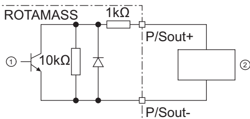
Fig. 43: Raccordement en série de la sortie d'impulsions ou d'état passive avec amplificateur de commutation
