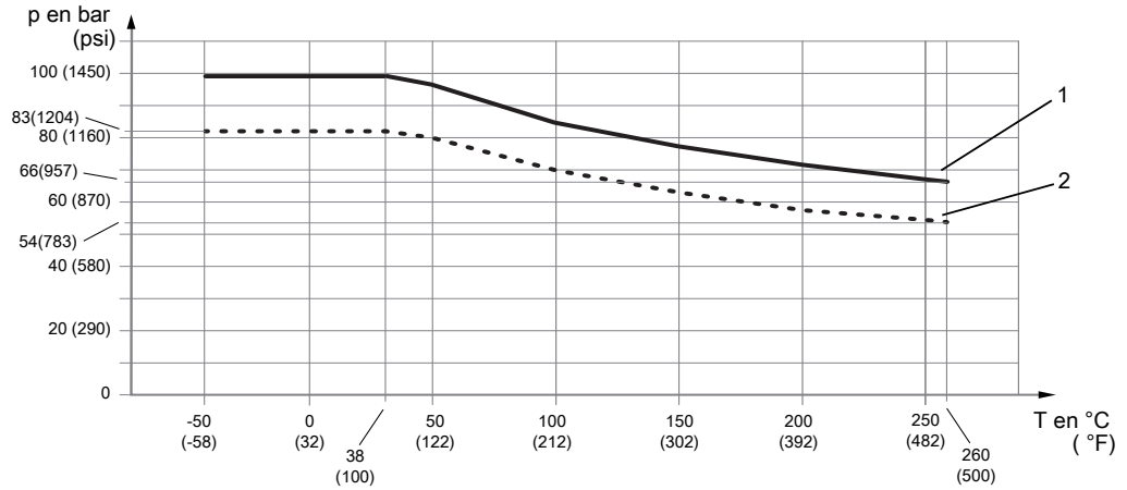
Fig. 14: Pression de service admissible en fonction de la température du raccordement process
