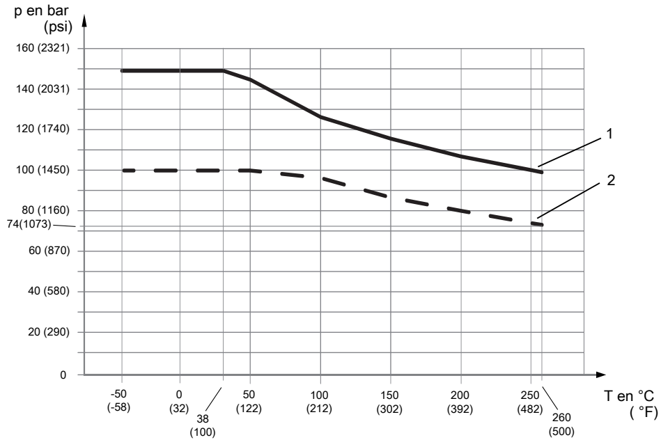
Fig. 15: Pression de service admissible en fonction de la température du raccordement process
