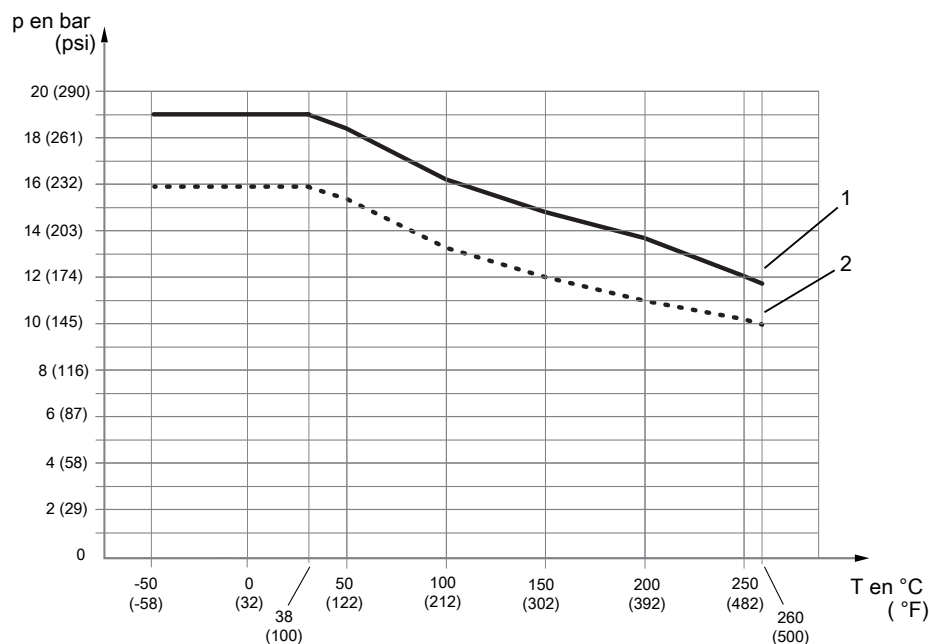
Fig. 12: Pression de service admissible en fonction de la température du raccordement process
