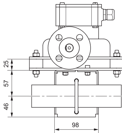
Fig. 28: Dimensions en mm : dispositif de fixation option PD pour Nano
