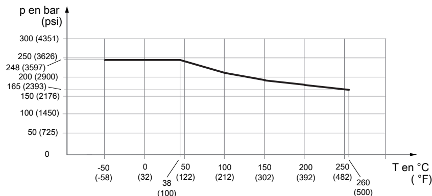
Fig. 16: Pression de service admissible en fonction de la température du raccordement process
