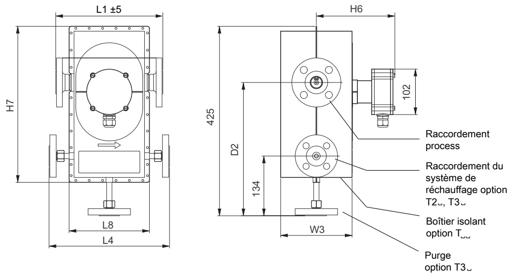
Fig. 27: Dimensions en mm : variante avec boîtier isolant
