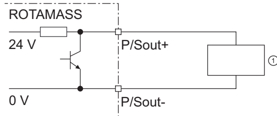
Fig. 40: Sortie d'état active P/Sout avec résistance interne pull-up
