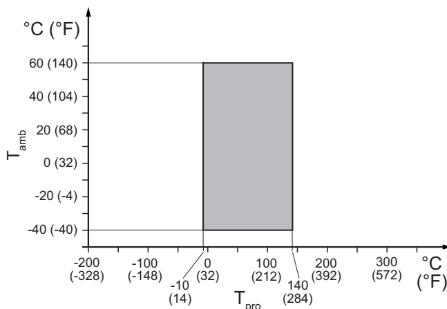
Fig. 17: Températures ambiantes et de service admissibles du fluide à mesurer, type intégral pour raccordement process HS4 et HS8
