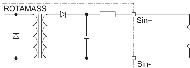
Fig. 39: Raccordement de l'entrée d'état
