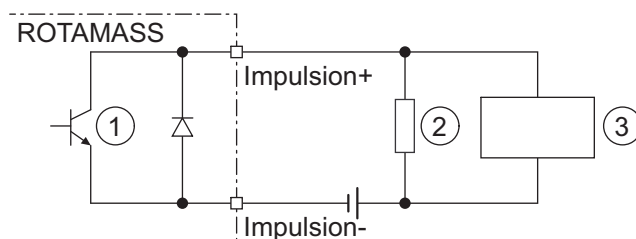
Fig. 41: Raccordement de sortie d'impulsion passive avec compteur électronique
