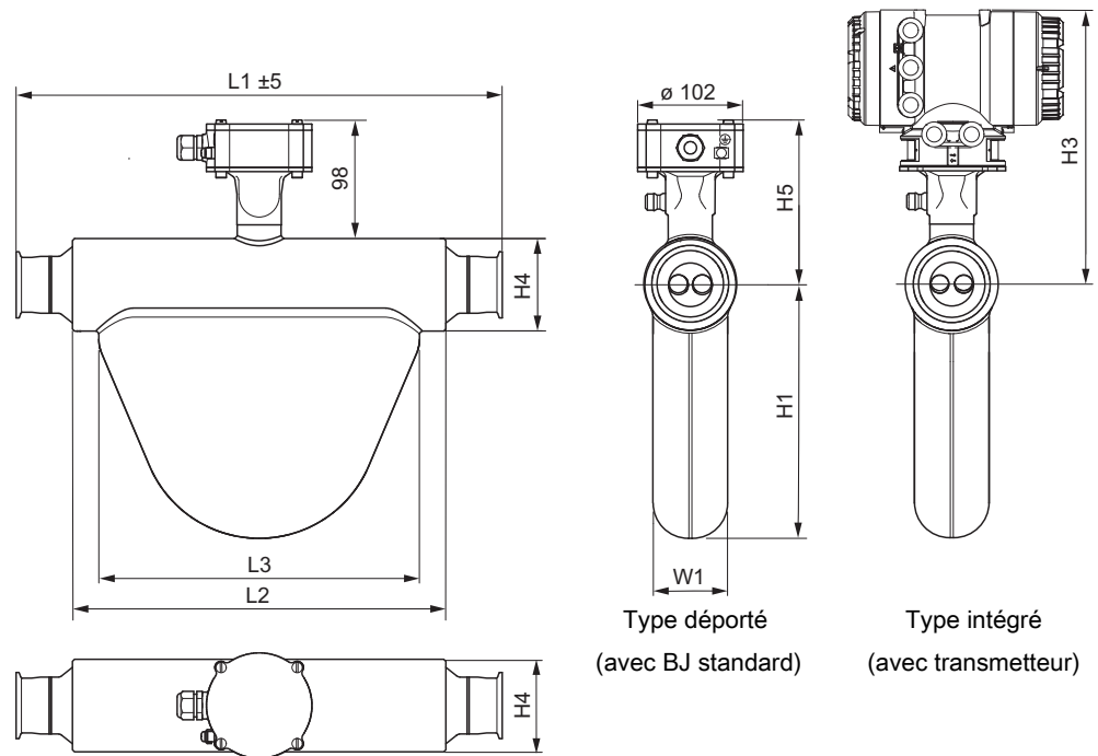
Fig. 21: Dimensions en mm
