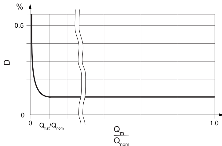
Fig. 9: Dépendance schématique de la précision de mesure du débit massique
