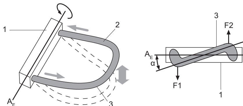
Fig. 2: Forces de Coriolis et déformations des tubes de mesure
