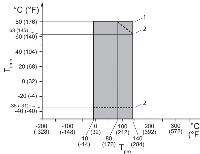
Fig. 19: Température de service du fluide à mesurer et température ambiante admissibles, type déporté pour raccordement process HS4 et HS8
