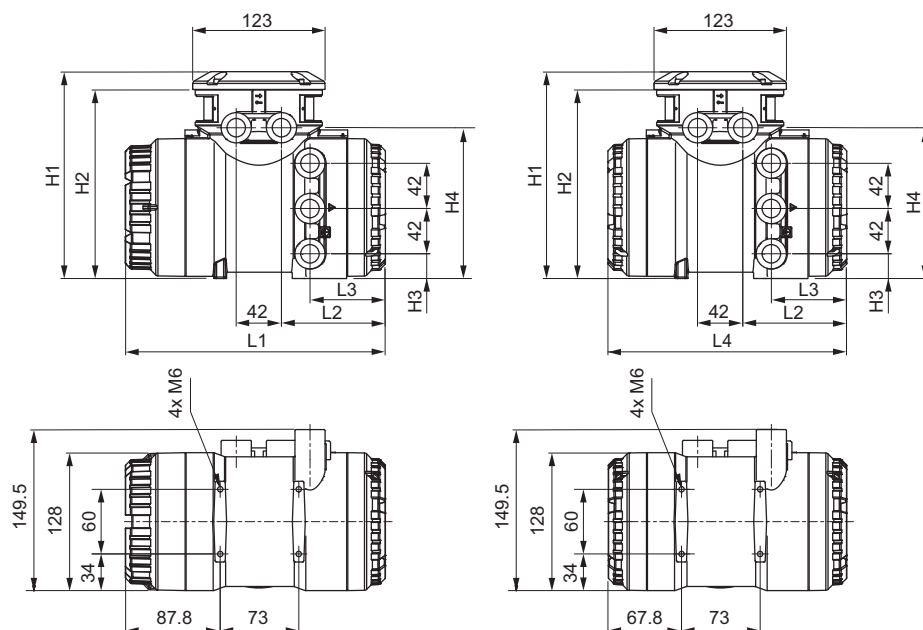
Fig. 22: Dimensions du transmetteur en mm (à gauche : transmetteur avec écran, à droite : transmetteur sans écran)
