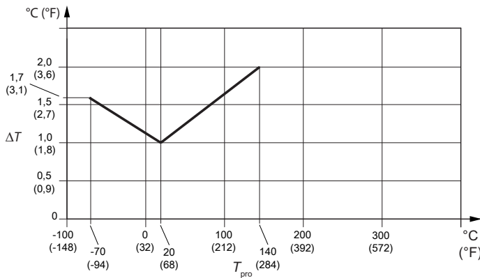
Fig. 10: Représentation de la précision de mesure de la température
