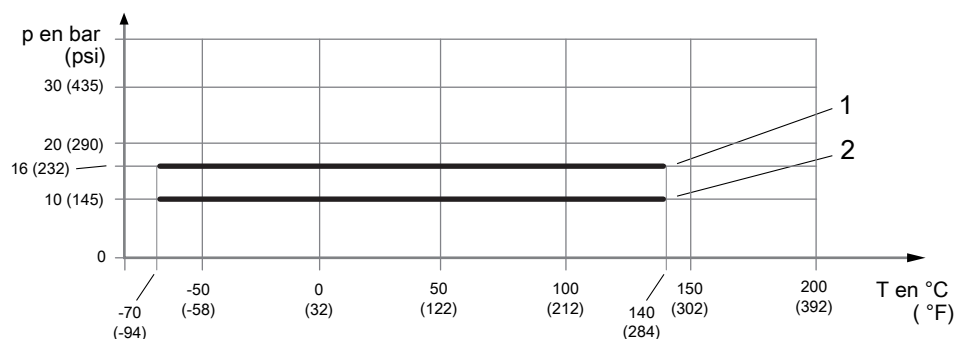
Fig. 15: Pression de service admissible en fonction de la température du raccordement process
