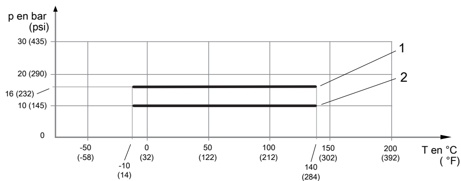
Fig. 14: Pression de service admissible en fonction de la température du raccordement process
