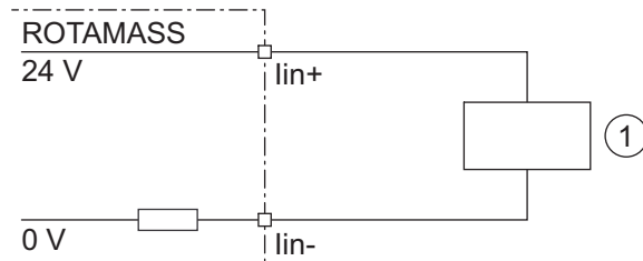
Fig. 37: Raccordement d'un appareil externe avec sortie de courant passive
