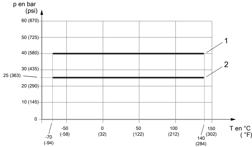
Fig. 12: Pression de service admissible en fonction de la température du raccordement process
