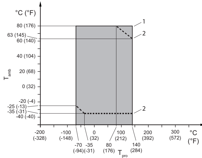
Fig. 18: Température de service du fluide à mesurer et température ambiante admissibles, type déporté pour raccordement process HS2 et HS9
