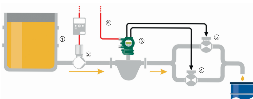
Fig. 44: Mode en deux étapes (le schéma ci-dessus illustre les fonctionnalités fondamentales pour l'une des nombreuses possibilités de combinaisons)
