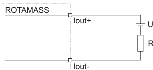
Fig. 26: Raccordement de la sortie de courant passive I out
