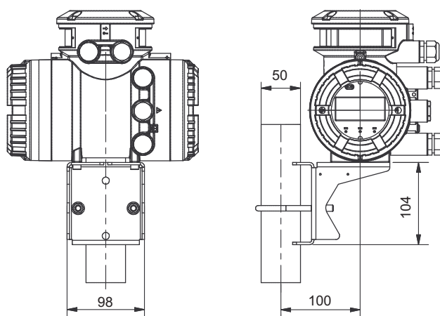
Fig. 23: Dimensions du transmetteur en mm, fixé à l'étrier de maintien
