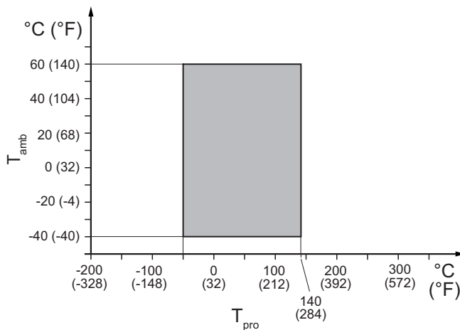
Fig. 16: Températures ambiantes et de service admissibles du fluide à mesurer, type intégral pour raccordement process HS2 et HS9
