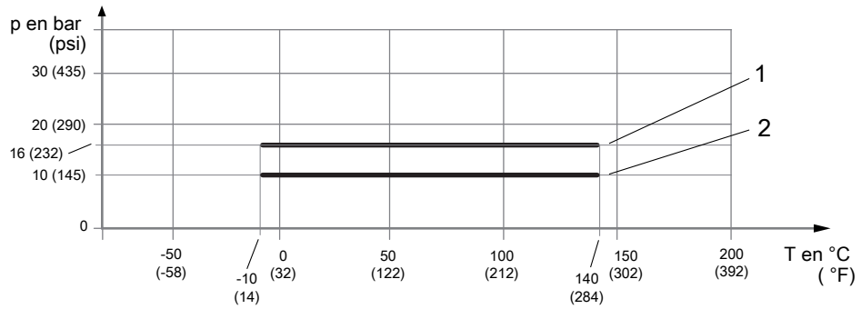
Fig. 13: Pression de service admissible en fonction de la température du raccordement process
