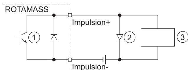
Fig. 42: Raccordement de sortie d'impulsion passive avec compteur électromécanique
