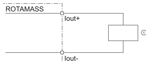
Fig. 24: Raccordement de la sortie de courant active HART I out
