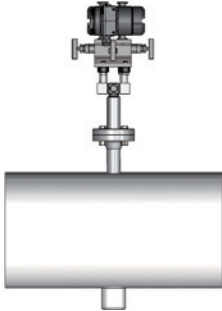
Flanschanschluss (DF12 / DF25 / DF44)
