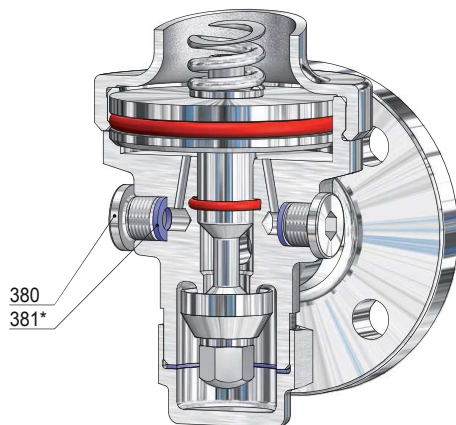
Alésage pour manomètre G 1/4
