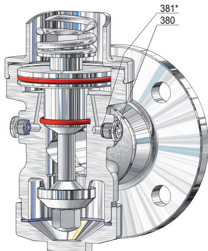
Alésage pour manomètre G ¼
