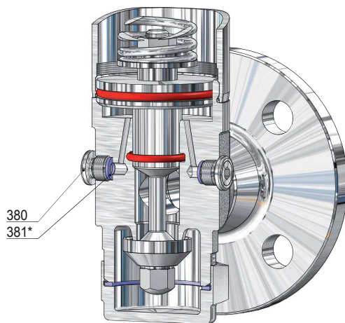
Alésage pour manomètre G 1/4
