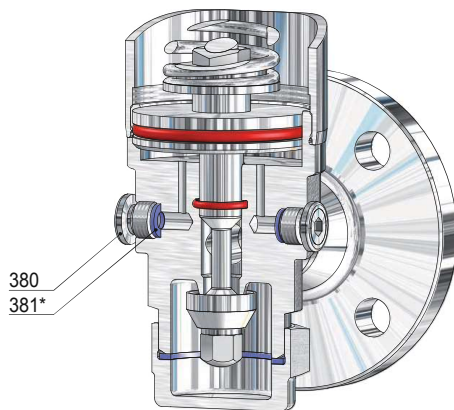
Alésage pour manomètre G ¼
