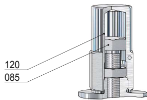
Soupape à coiffe (Option: AC)
