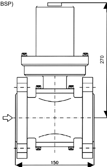
PR50: DN50 / PN40, 2" / 150 lbs
